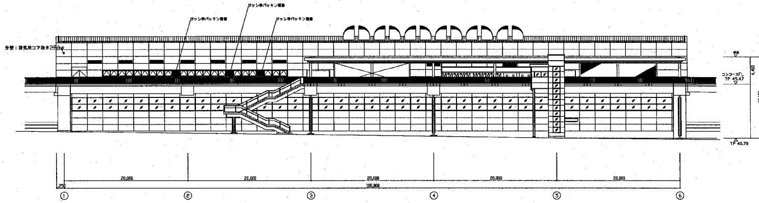
南立面図 1/200
