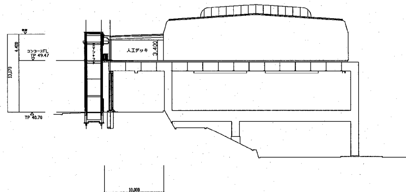
断面図 1/200
