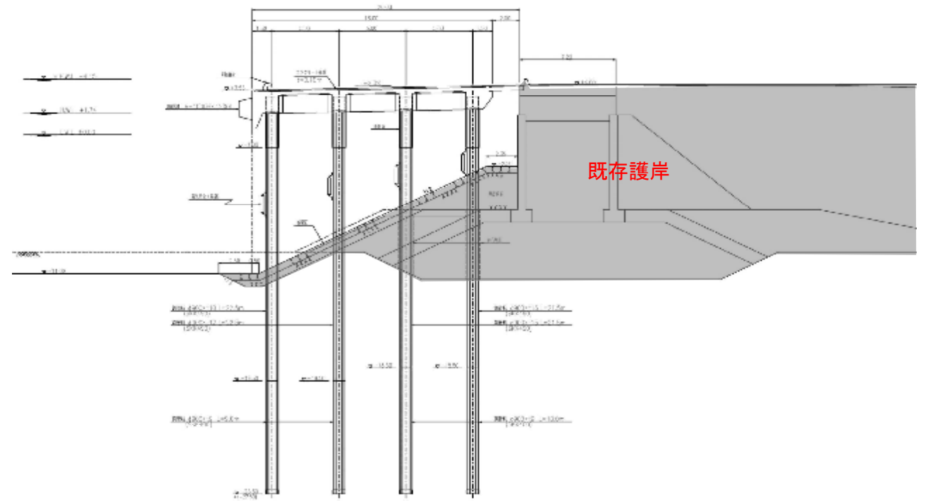
標準断面図
