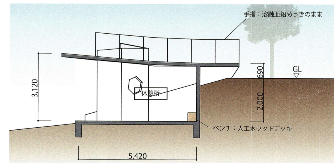
A-A 断面図 S=1/100
