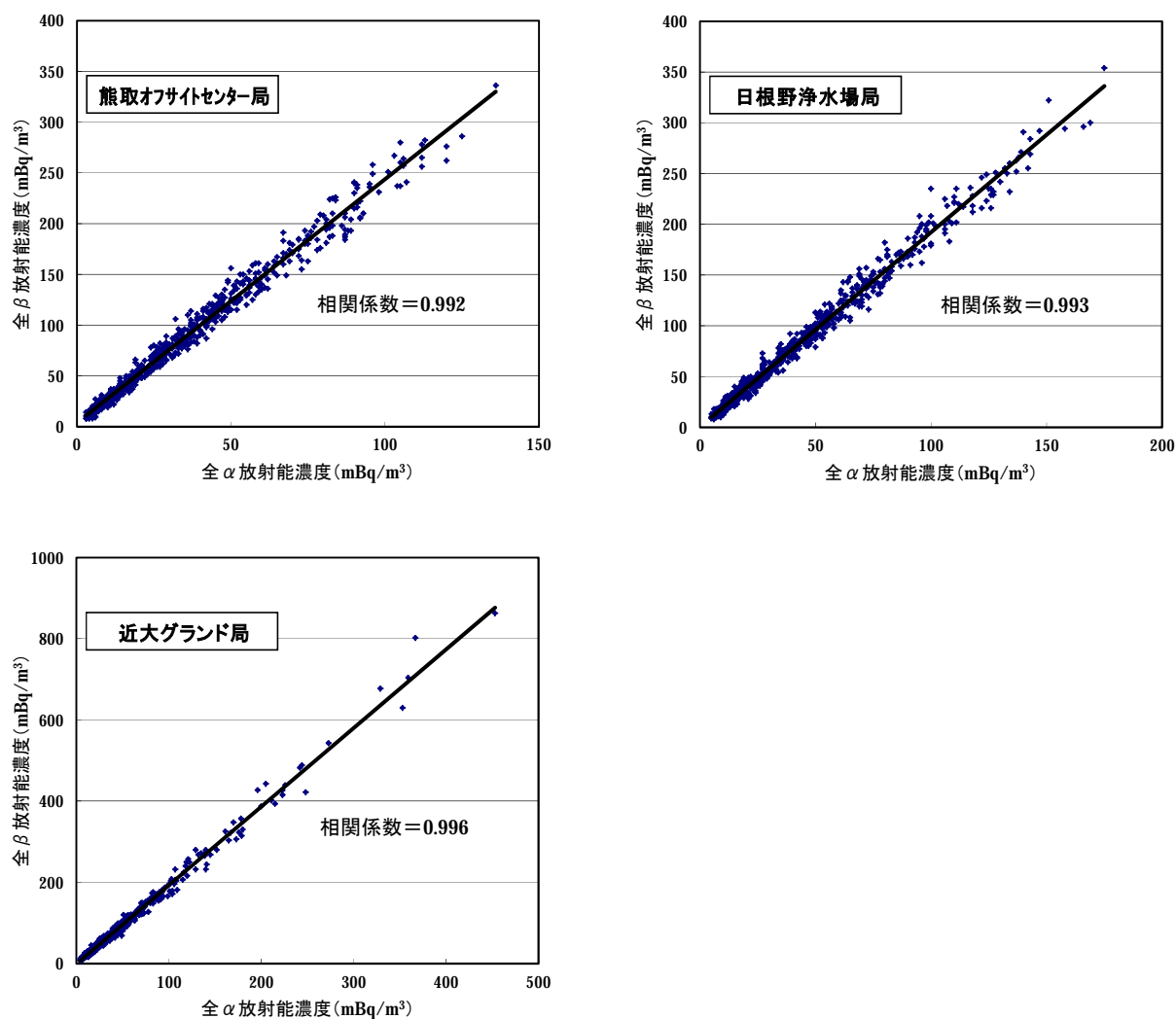
図Ⅲ-4 大気浮遊じん中全 \alpha 放射能濃度及び全 \beta 放射能濃度の相関関係
