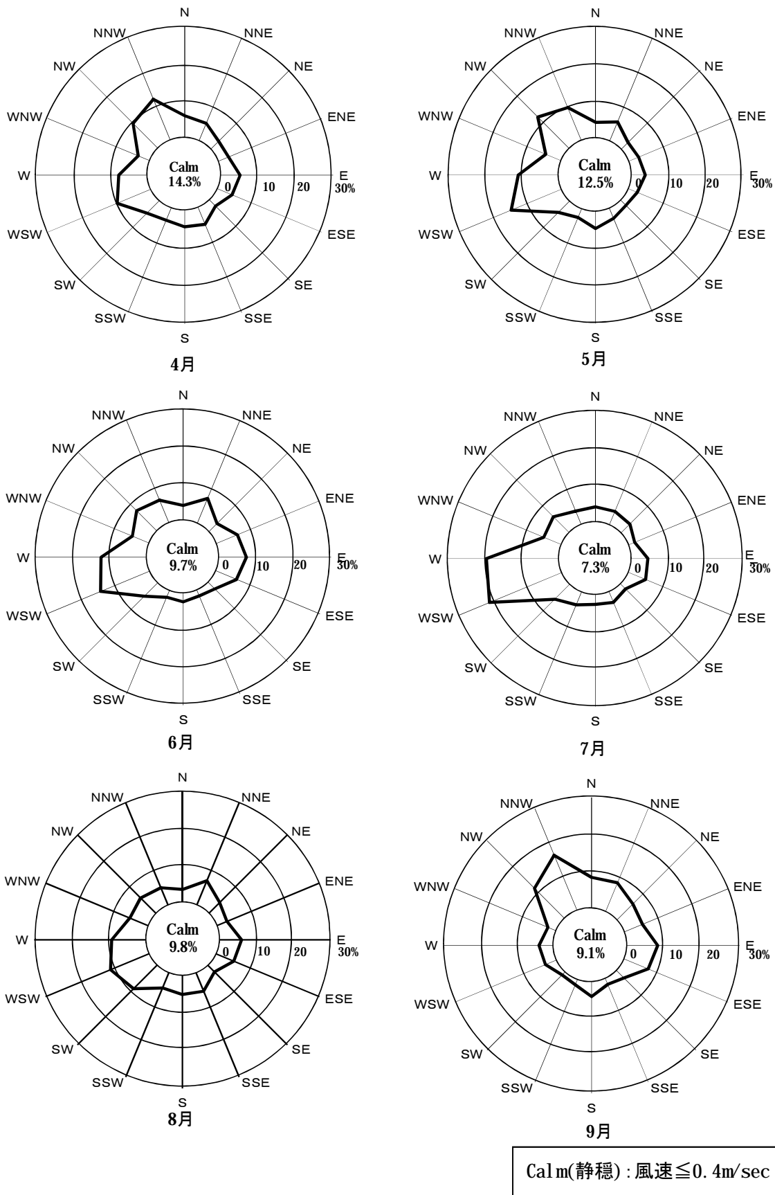
図Ⅲ-7 風配図 (近畿大学グラウンド局)
