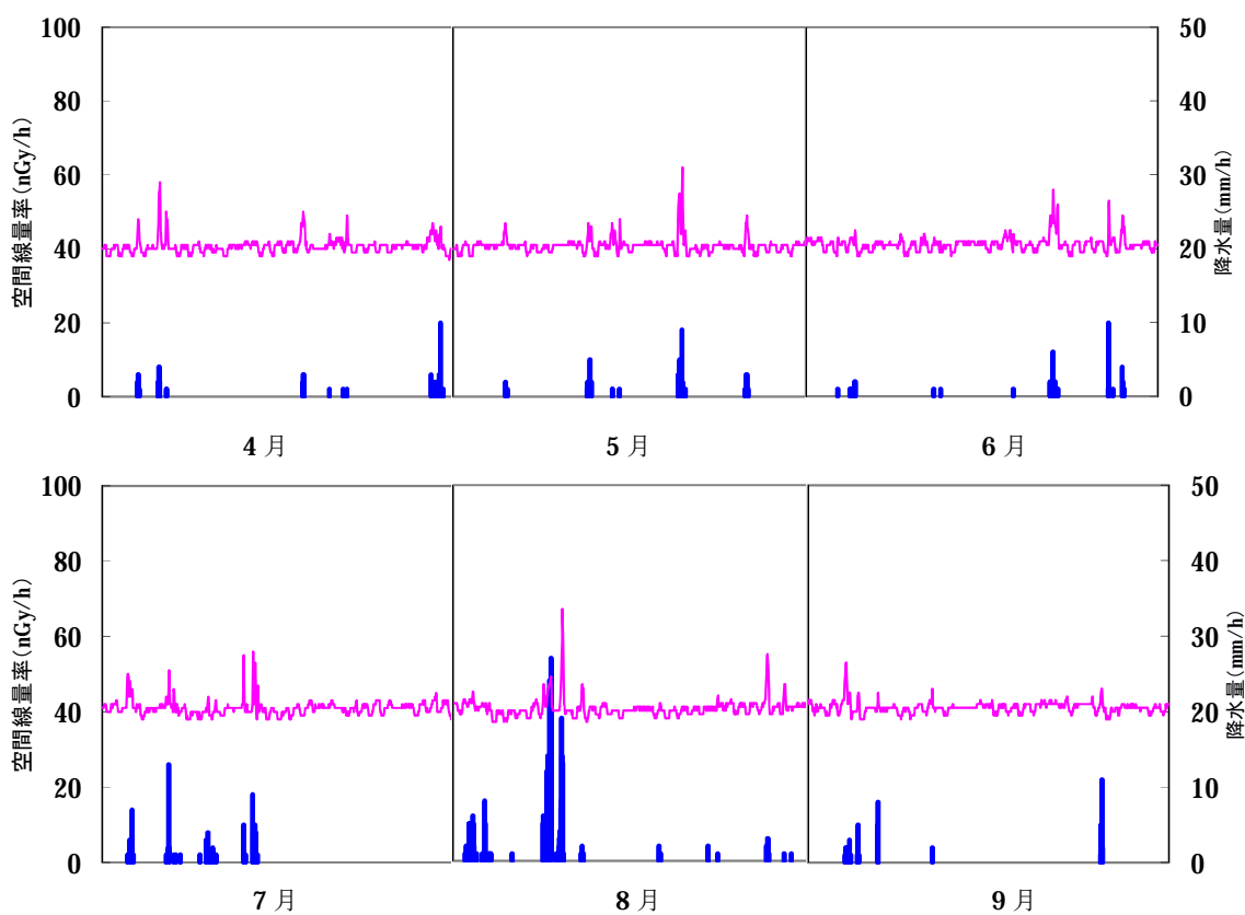
図Ⅲ-2 低線量トレンド（日根野浄水場局）
