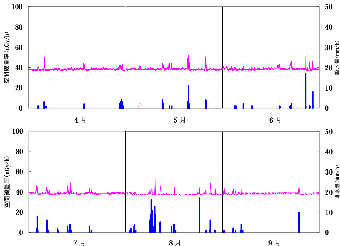
図Ⅲ-3 低線量トレンド（近畿大学グラウンド局）
