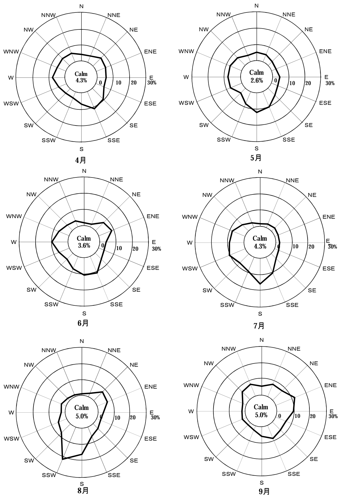
図III-6 風配図 (日根野浄水場局)
