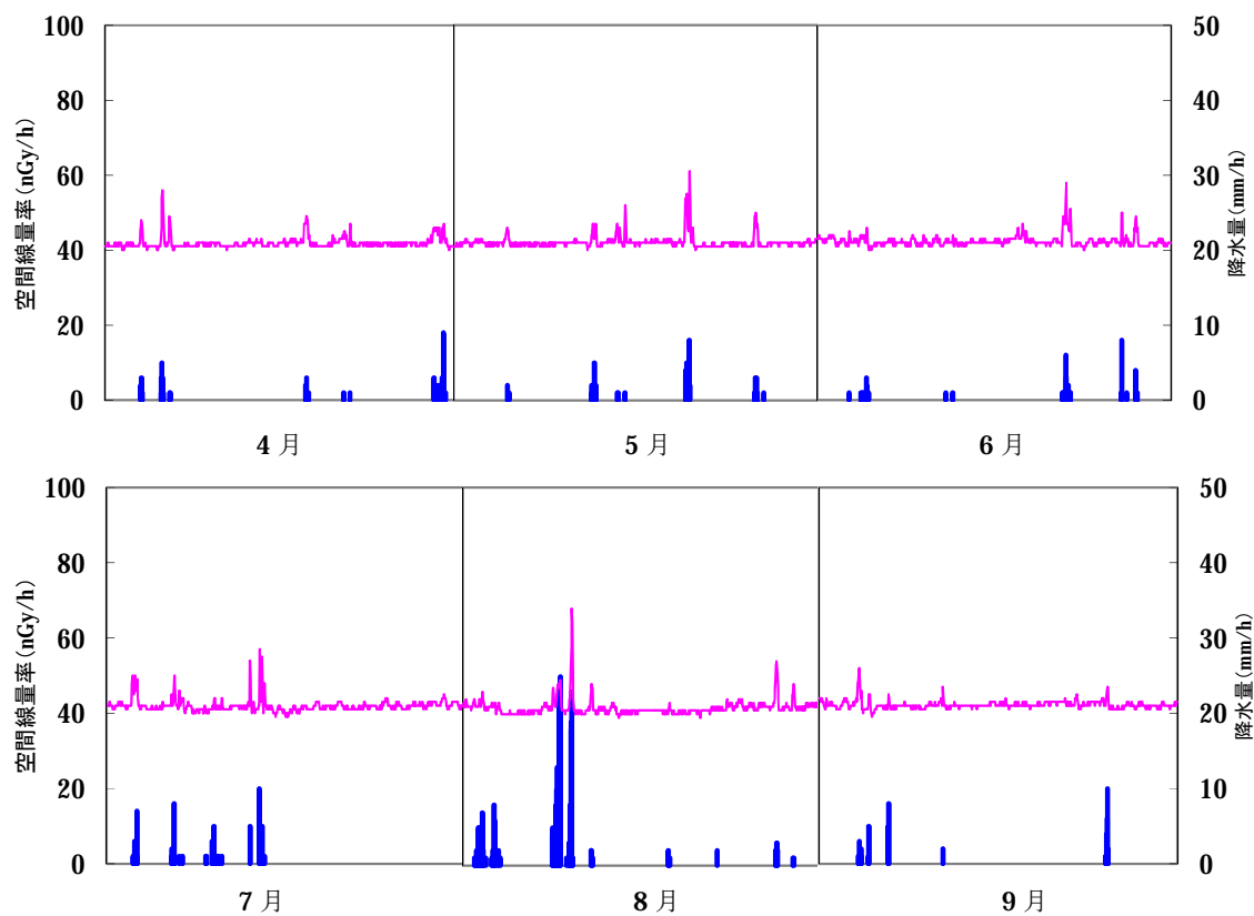
図Ⅲ-1 低線量トレンド（熊取オフサイトセンター局）
