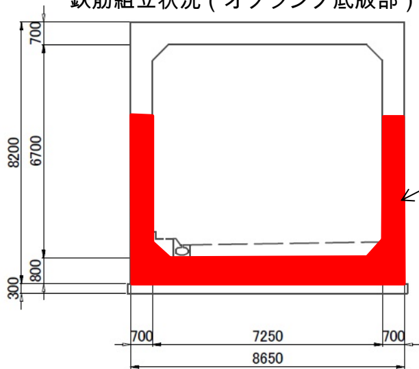
鉄筋組立状況 (オフランプ底版部)
