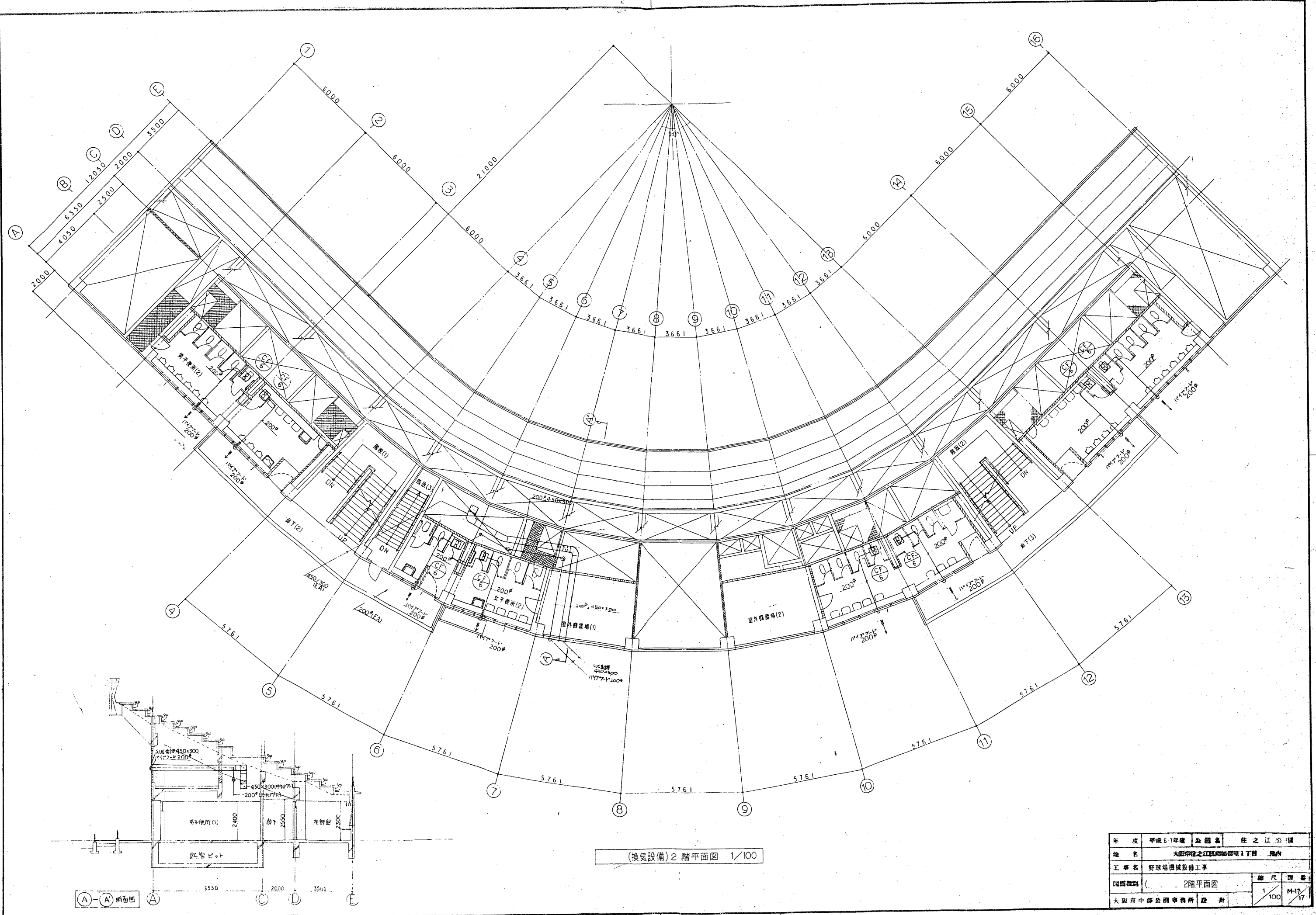
②住之江公園主要建物図面 (野球場2F)
