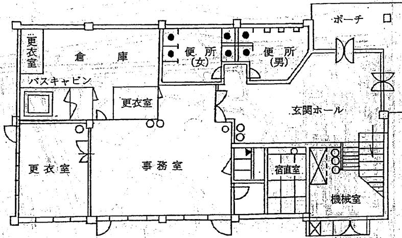
1階平面図
