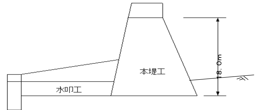
標準断面図
