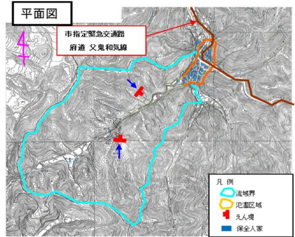
平面図
