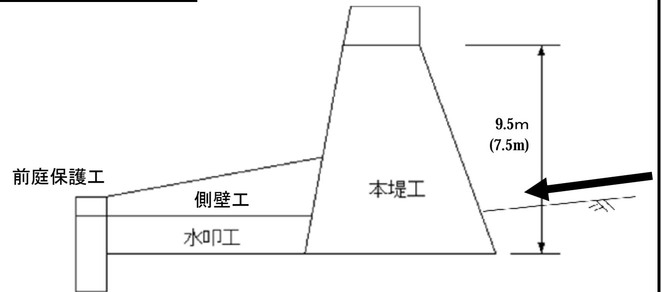
標準断面図
