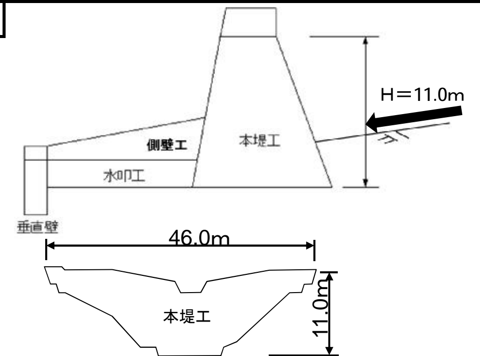
標準断面図
