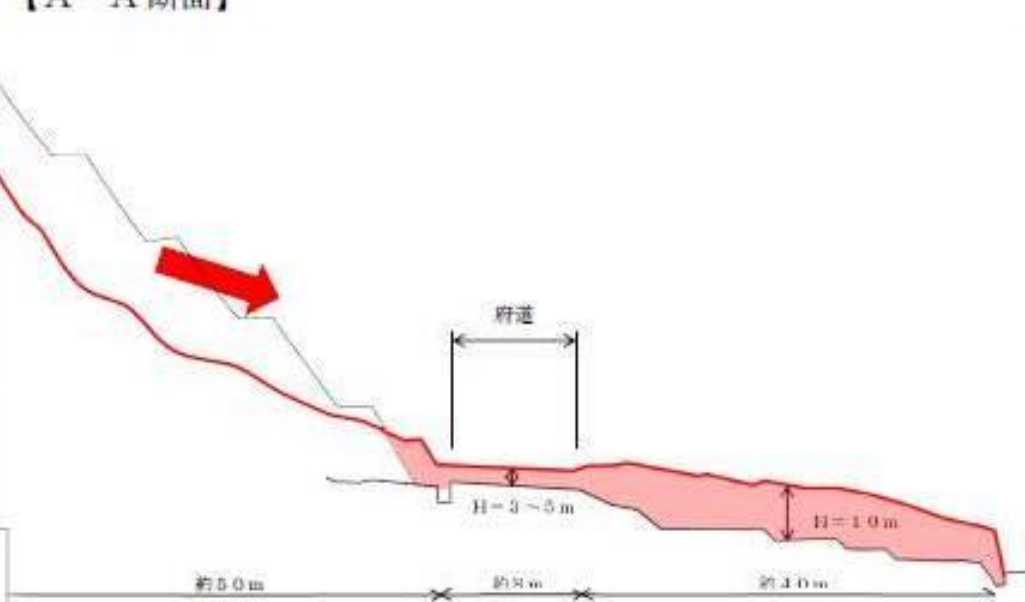
【A-A'断面】
