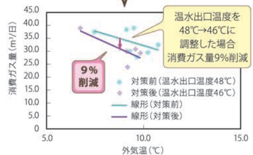
【温水出口温度の変化による外気温度と消費ガス量の関係】
