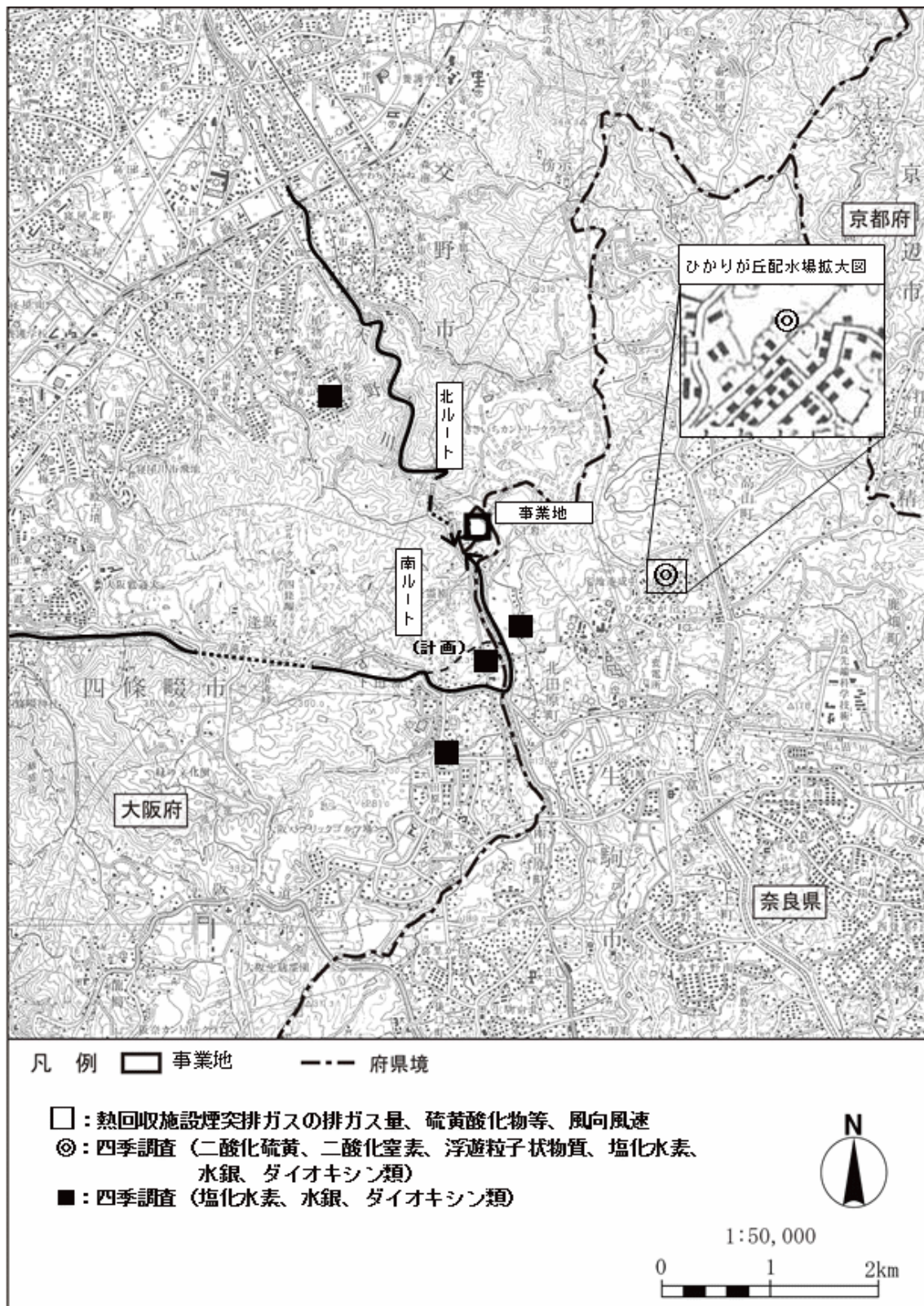
図1 供用時の事後調査地点 (大気質、気象)
