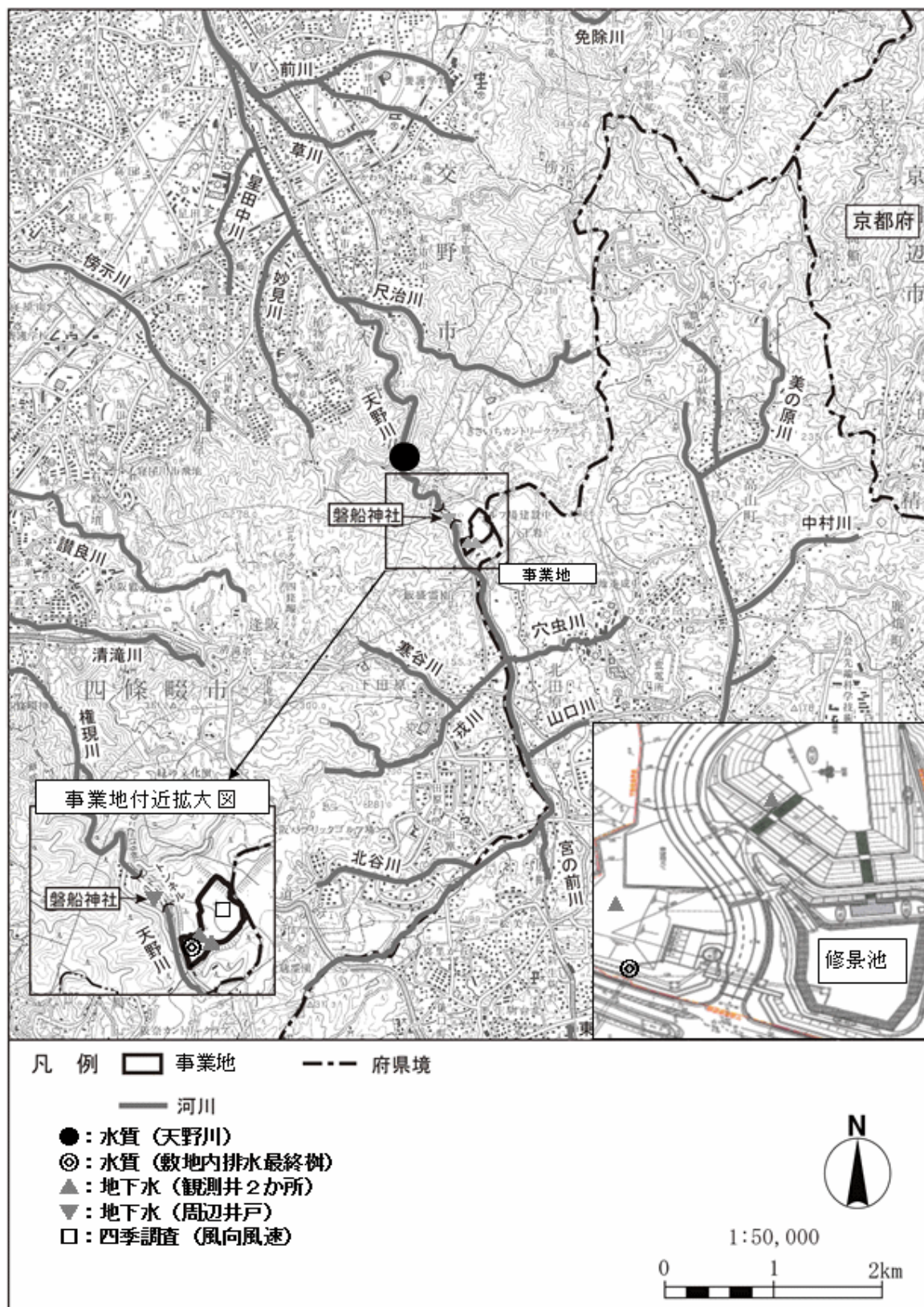
図2 供用時の事後調査地点 (水質、地下水)
