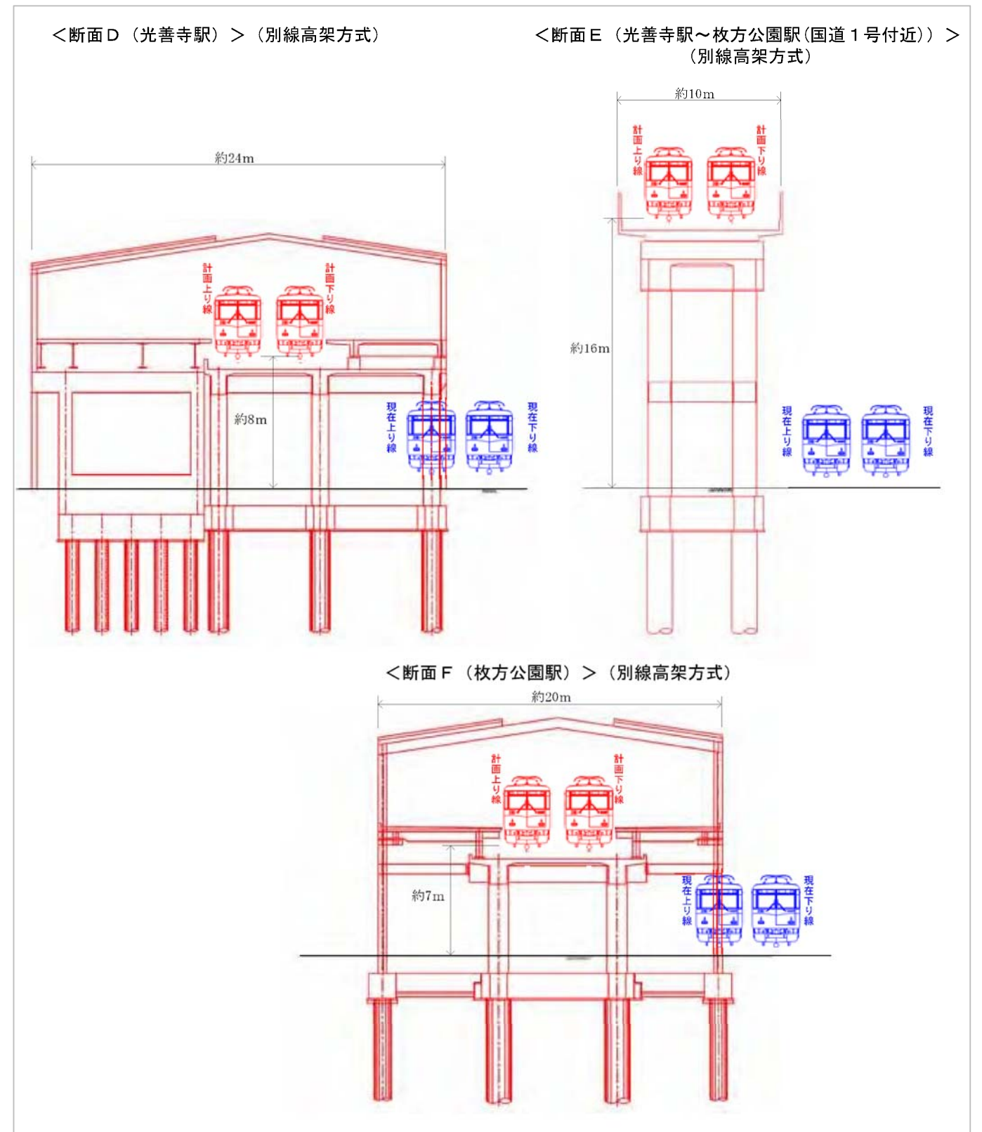
図 1.2(2) 高架化の概要 (断面D~F)
