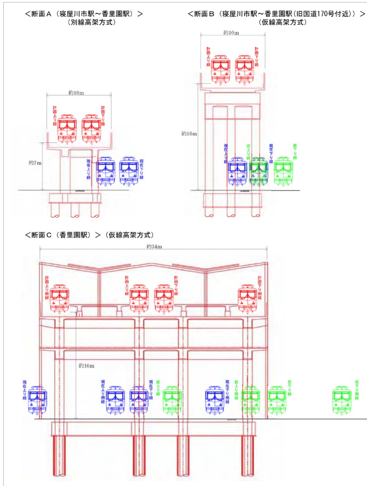
図 1.2(1) 高架化の概要 (断面A~C)
