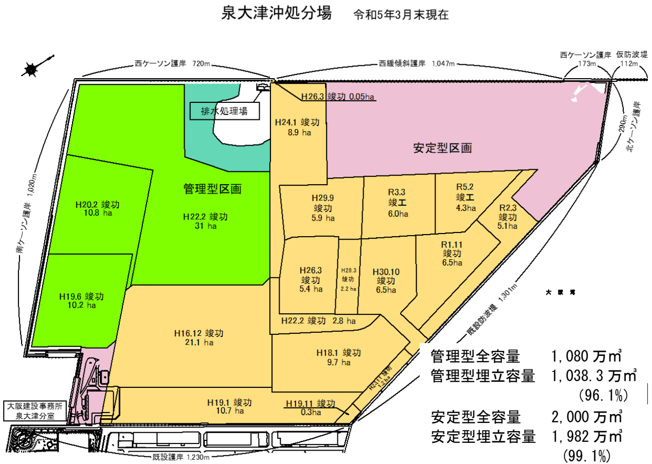
図2-2-4 埋立の進捗状況(令和5年3月末現在)
