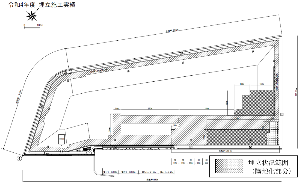
図2-1-5 埋立の進捗状況(令和5年3月末現在)
