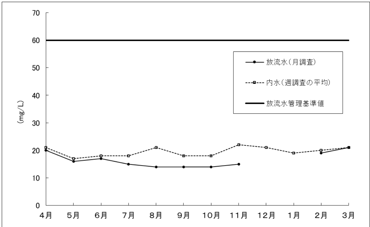
図 3-2-9 管理型区画内水及び放流水 COD の経月変化
