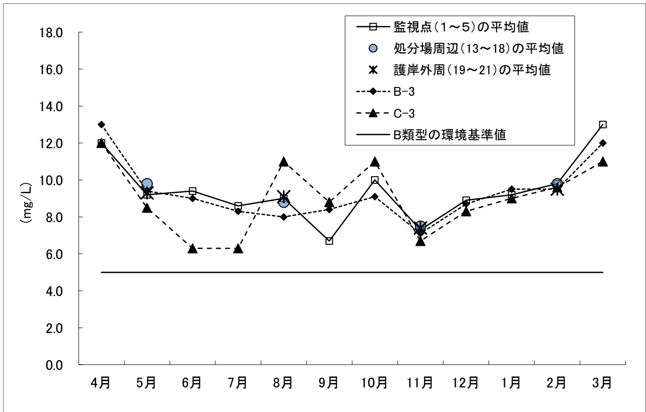
図 3-1-4 DO (上層) の経月変化
