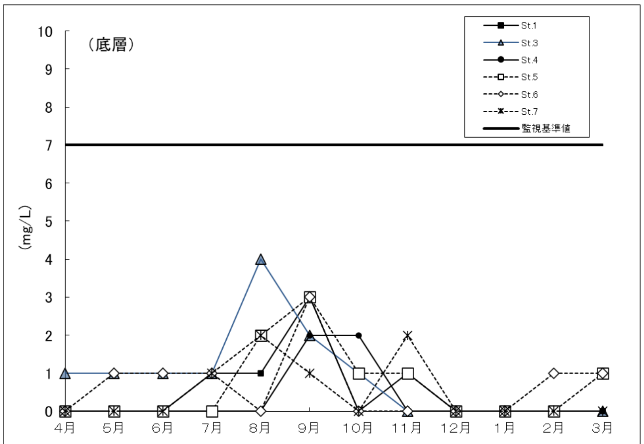
図 3-2-3 基本監視点における FSS の経月変化
