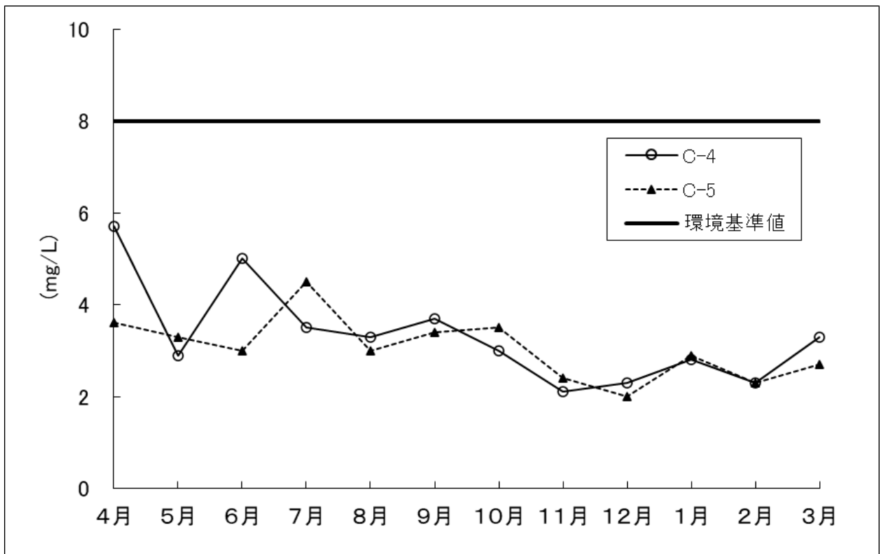
図 3-2-8 COD (表層) の経月変化 (大阪府による周辺海域 (C海域: 2点) の月調査結果)
