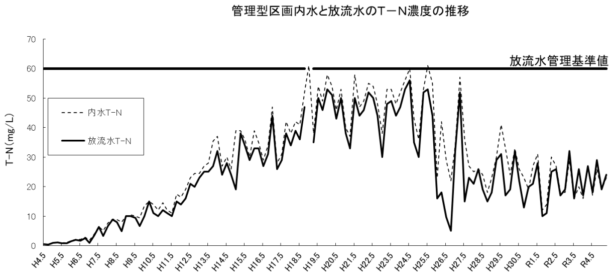
図 3-2-10 管理型区画内水及び放流水の水質の経年変化
