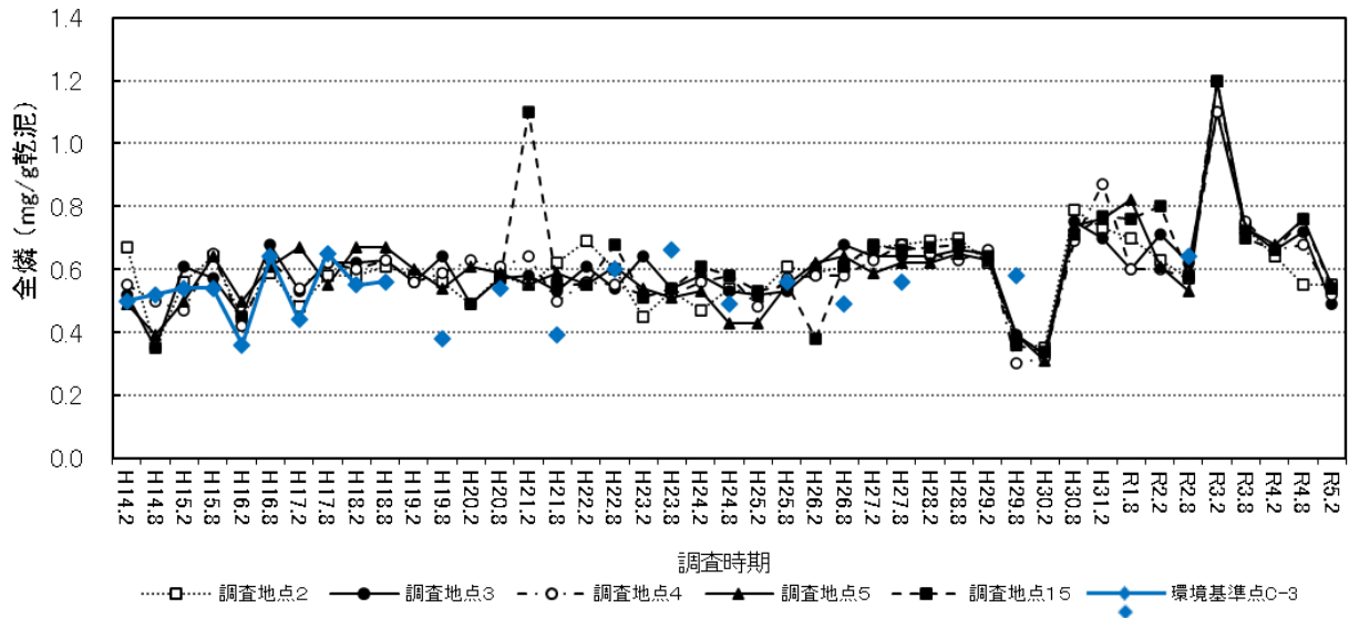
図 3-1-8(2) 底質調査結果の経年変化 (T-P)
