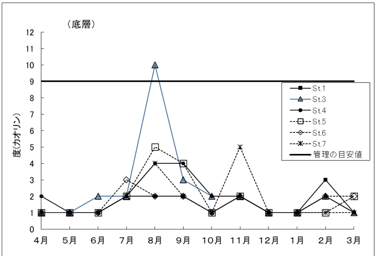
図 3-2-4 基本監視点における濁度の経月変化
