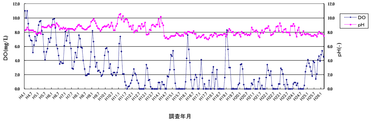
管理型区画内水のDOとpHの推移
