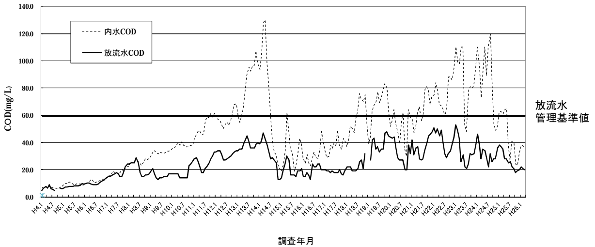
管理型区画内水と放流水のCODの推移
