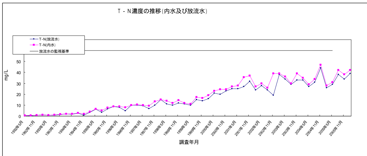
図 3 - 1 - 10 管理型内水及び放流水の経年変化
