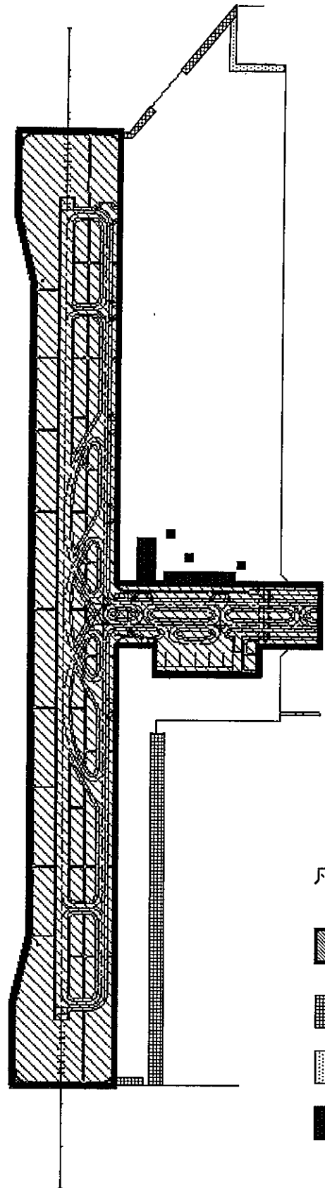
2期空港島建設工事概要図 (平成23年10月分)
