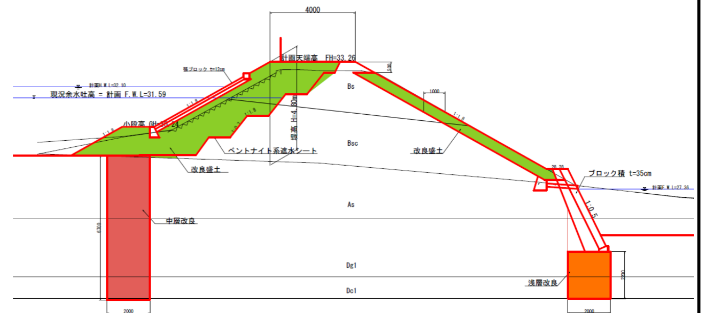
標準断面図
