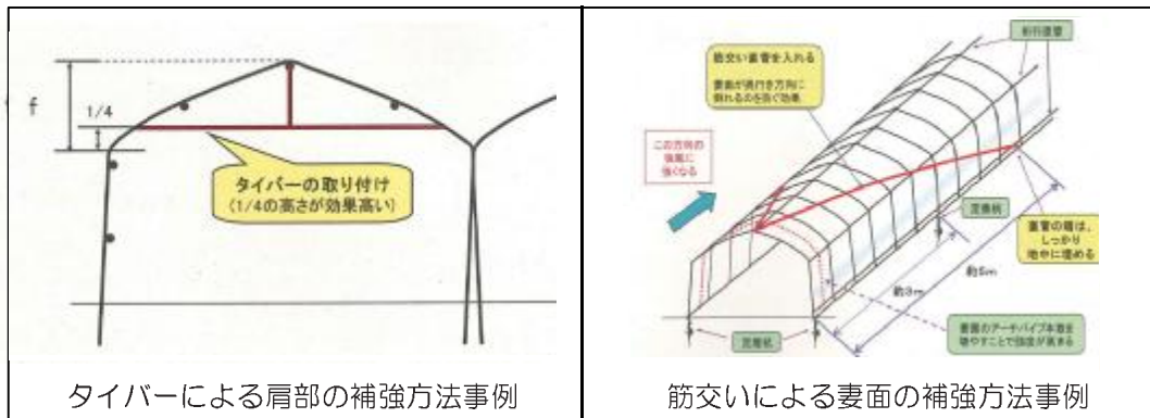
ハウス部位名称と補強策（農林水産省 HP の図を参考作成）
