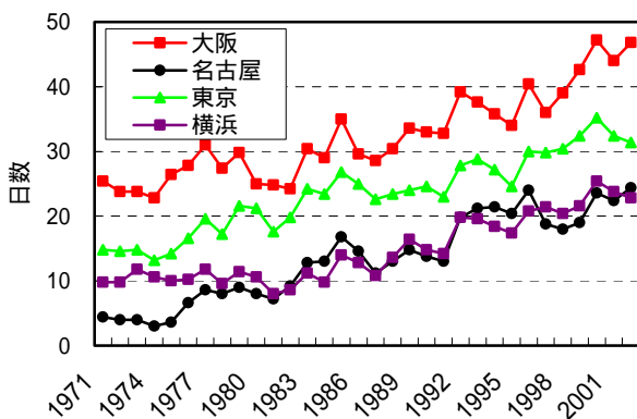
図 - 11 大都市における熱帯夜日数(5年移動平均)
