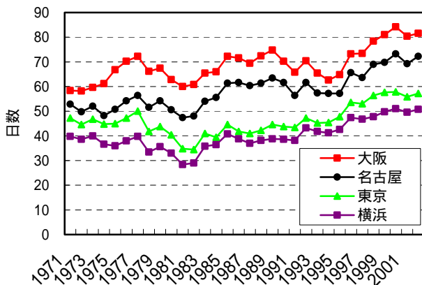
図 - 10 大都市における真夏日日数(5年移動平均)
