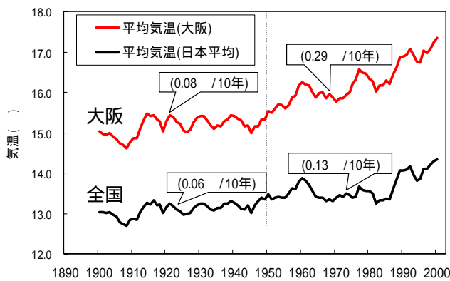
図 - 9 大阪・全国における年平均気温の推移
