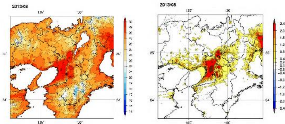
近畿地方を対象とした2013年8月の月平均気温の分布（°C）（左図）と 都市化の影響による月平均気温の変化（°C）（右図）
