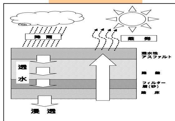
透水性舗装の仕組み
